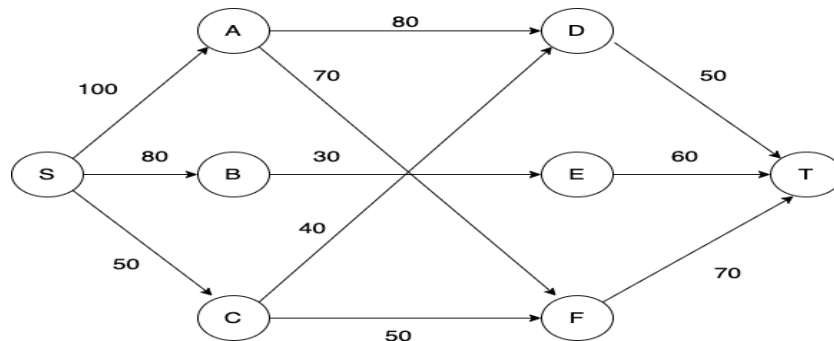
FIGURE 2 – Un réseau R = (V, E, C) . A \forall arc e \in E est affectée sa capacité c_e .
